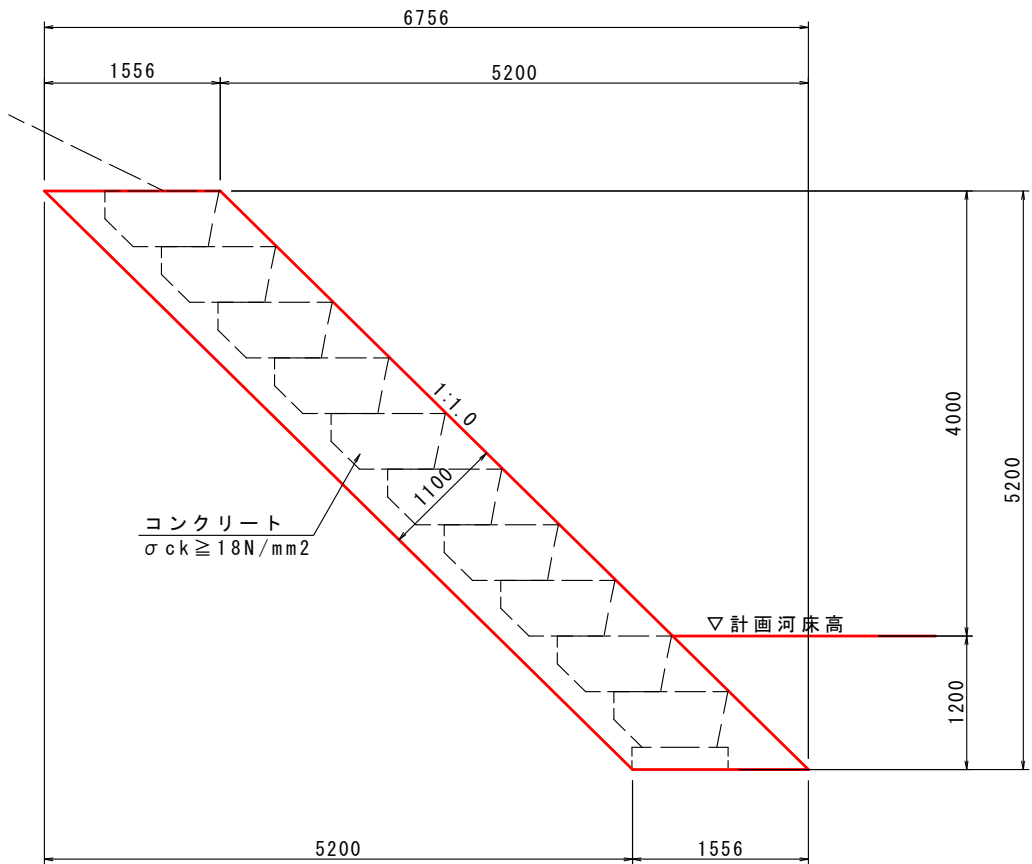
側面図
